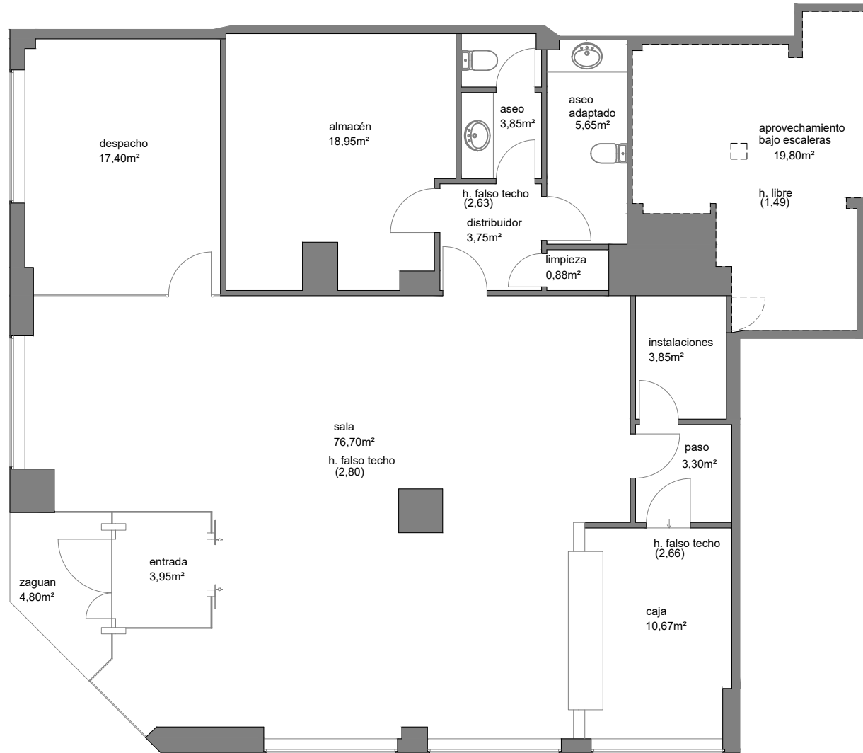
Bajo Esquina Edificio Alessa Escala (A4) 1:100
